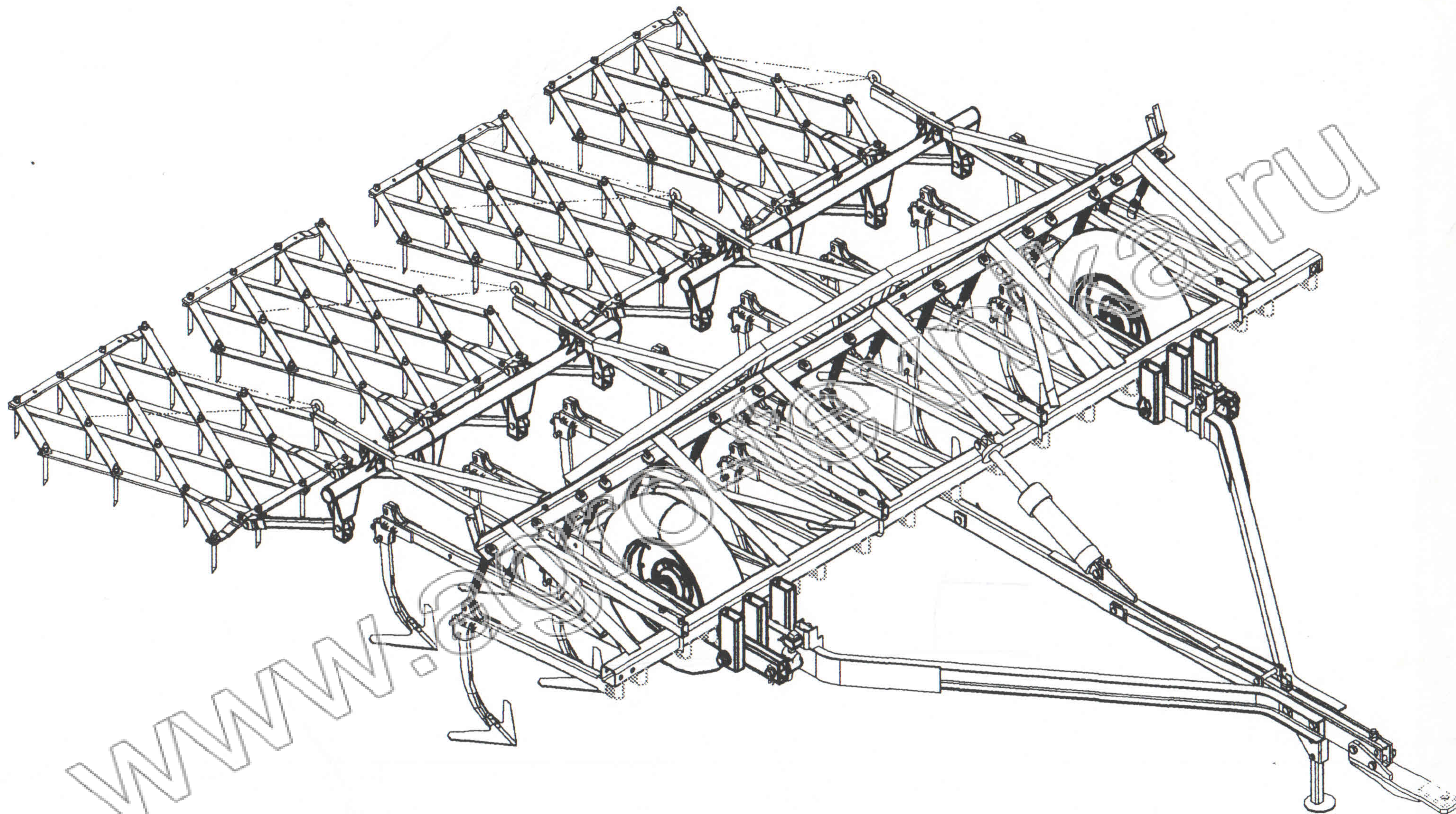
Общий вид Культиватор прицепной для сплошной обработки почвы КПС-4У "КОРММАШ"
