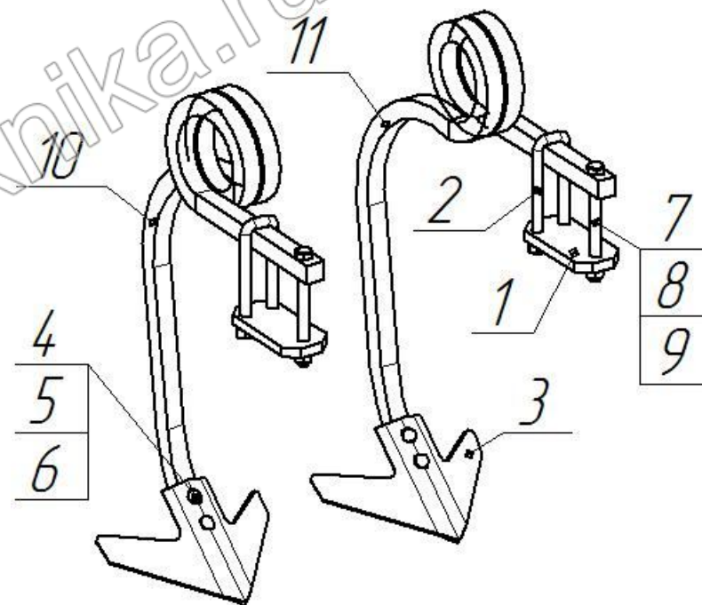
Рисунок 2 – АКЧ-6 04.000 Стойка в сборе, АКЧ-6 04.000-01 Стойка в сборе 1 – АКЧ-6 04.401 Пластина, 2 – КЧ 01.00.004 Скоба, 3 – ЛС 00.402 Лапа стрелчатая, 4 – Болт М12х60.58 ГОСТ 7786-81, 5 – Гайка М12.5 ГОСТ 5915-70, 6 – Шайба 12.65Г ГОСТ 6402-70, 7 – Болт М16х180.88 ГОСТ 7798-70, 8 – Гайка М16.9 ГОСТ 5915-70, 9 – Шайба 16.65Г ГОСТ 6402-70, 10 – 315161 Стойка правая, 11 – 315171 Стойка левая.
