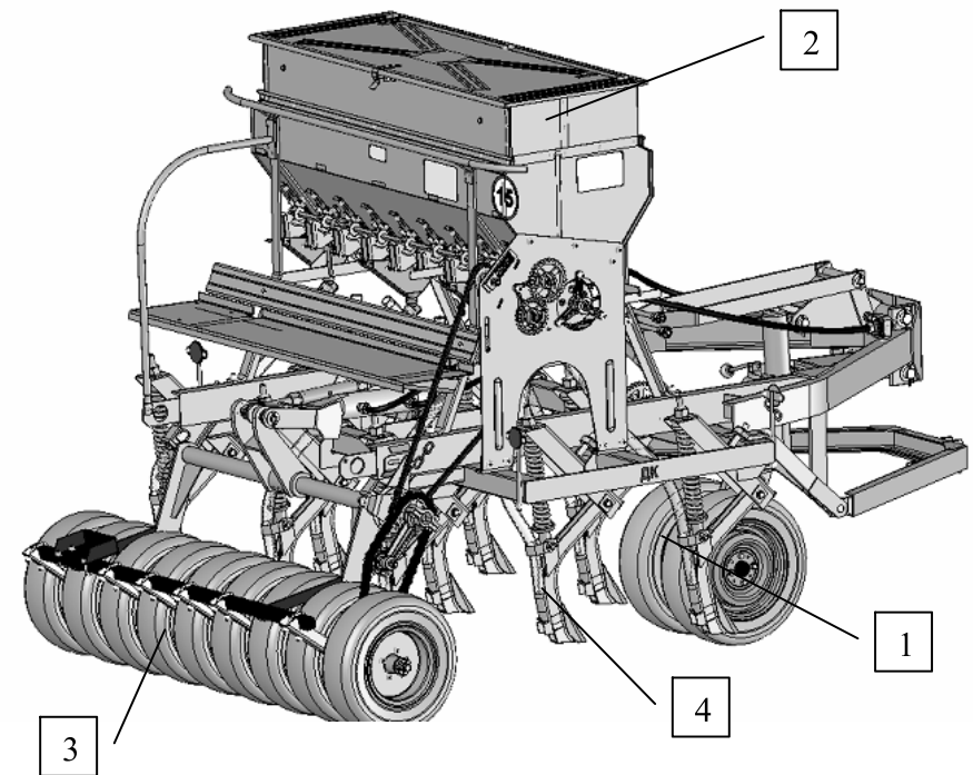
Рисунок 36- Сеялка СКП-2,13
