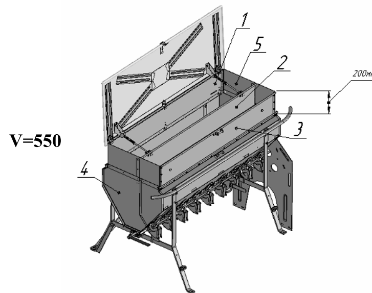
Рисунок 29- Ящик зернотуковый увеличенной ёмкости СКП 01.13.000А
