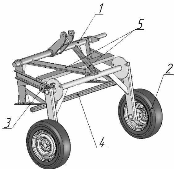
Рисунок 33- Задняя колёсная опора СКП-2,1К8
