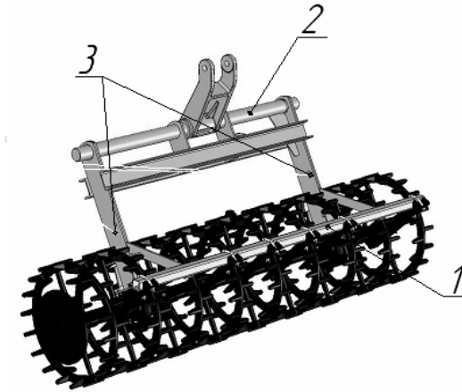
Рисунок 42 -Рамка с батареей катков.
