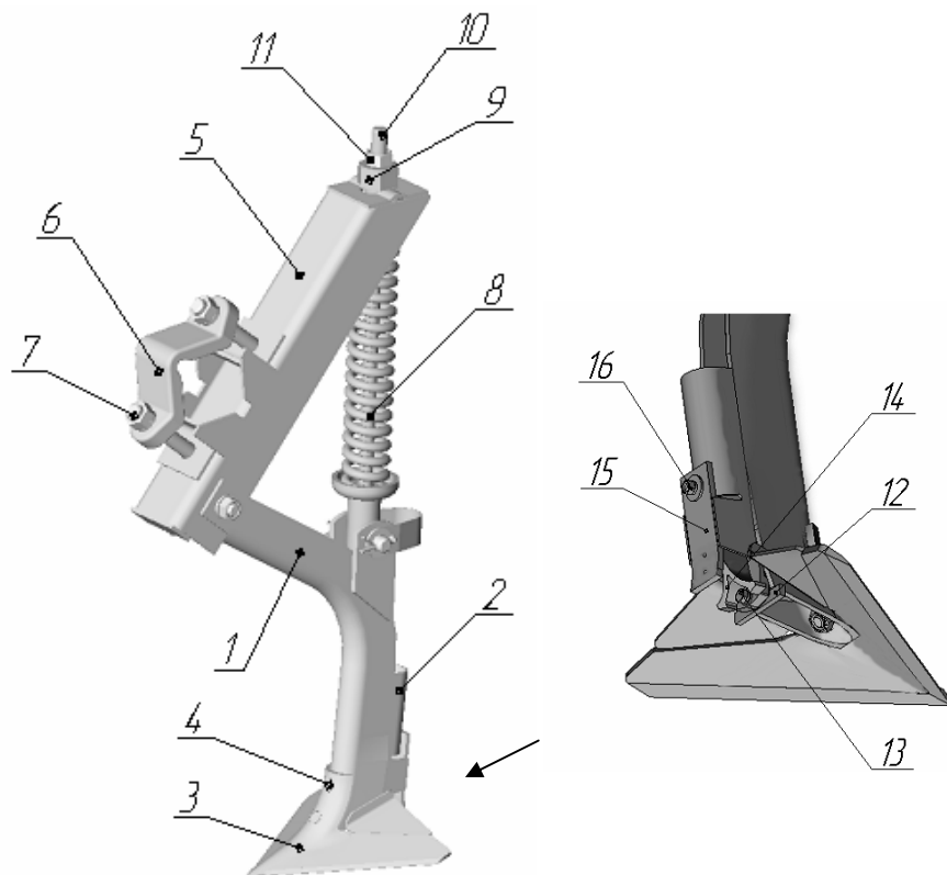
Рисунок 11- Рабочий орган (сошник) СКП 01.08.000Б
