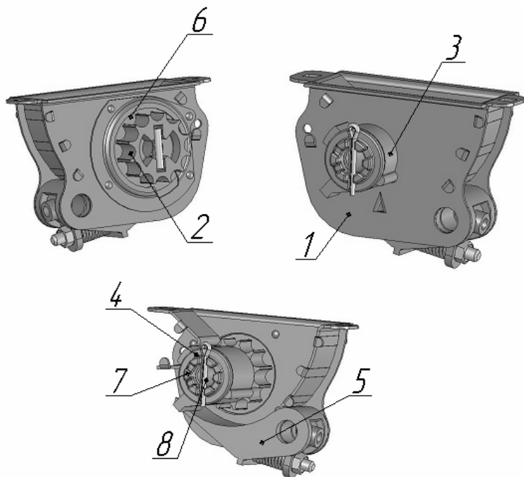
Рисунок 7- Зерновой высеваящий аппарат СКП 01.13.210
