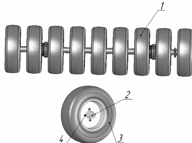
Рисунок 38- Батарея катков с пневмокатками СКП 01.23.000В
