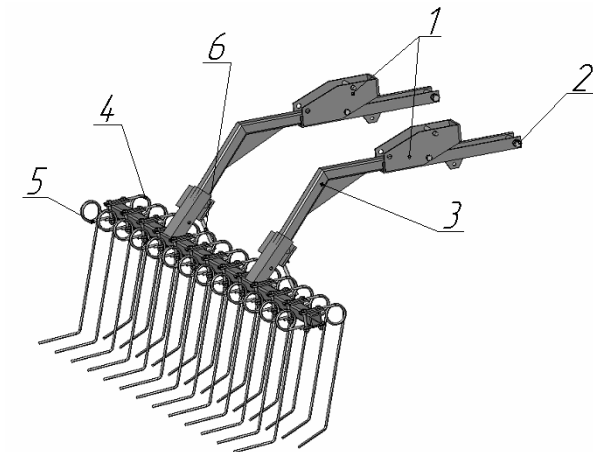
Рисунок 43- Борона пружинная СКП 01.39.000
