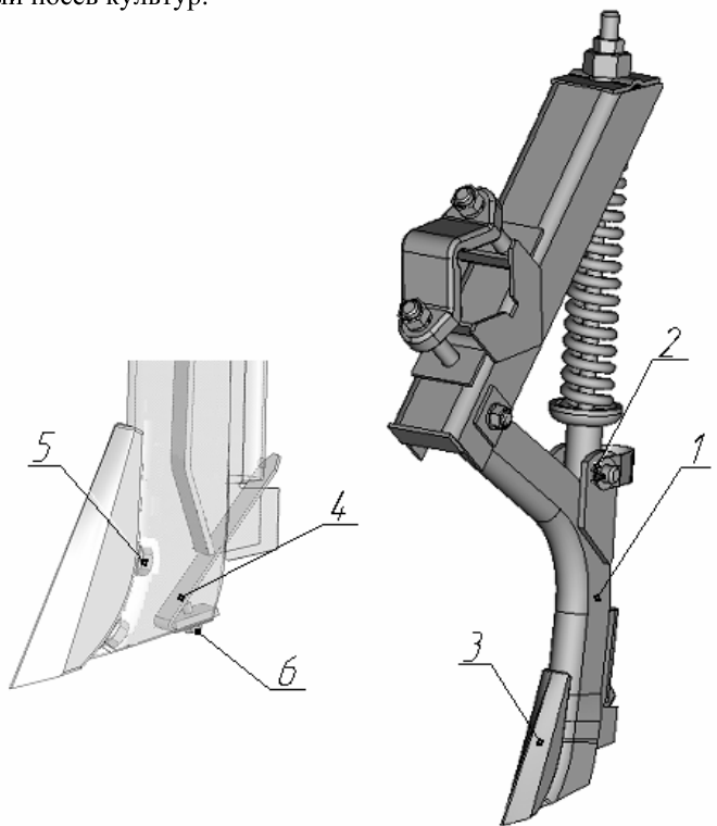
Рисунок 37- Сошник анкерный СКП01.08.000Д
