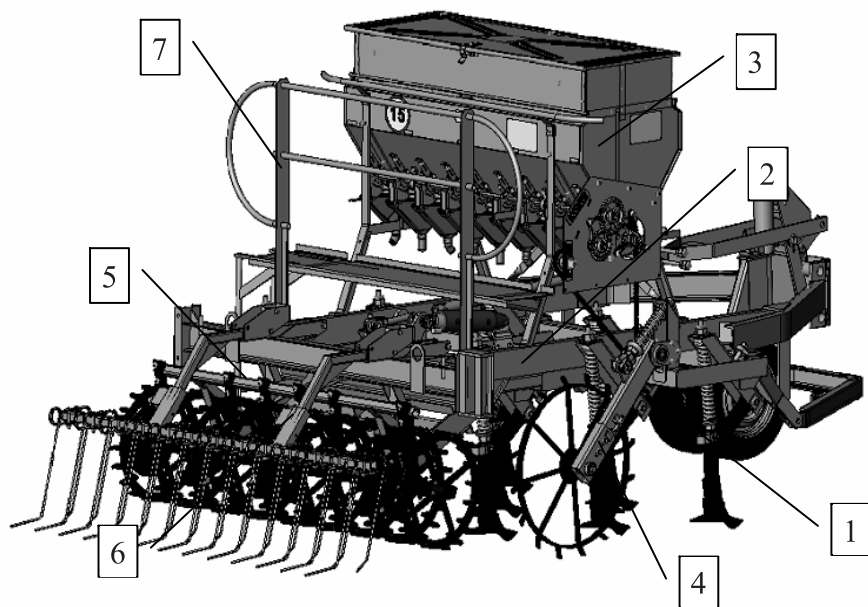
Рисунок 39-Сеялка СКП-2,1И
