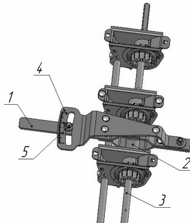
Рисунок 8- Регулятор нормы высева
