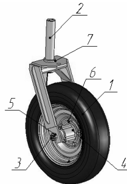
Рисунок 4- Опора передняя
