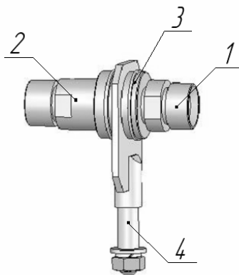
Рисунок 14 – Муфта разрывная
