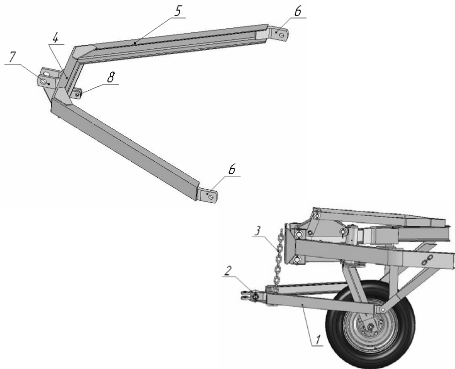
Рисунок 3- Устройство прицепное
