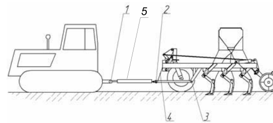
Рисунок 18- Схема соединения трактора с посевным комплексом.
