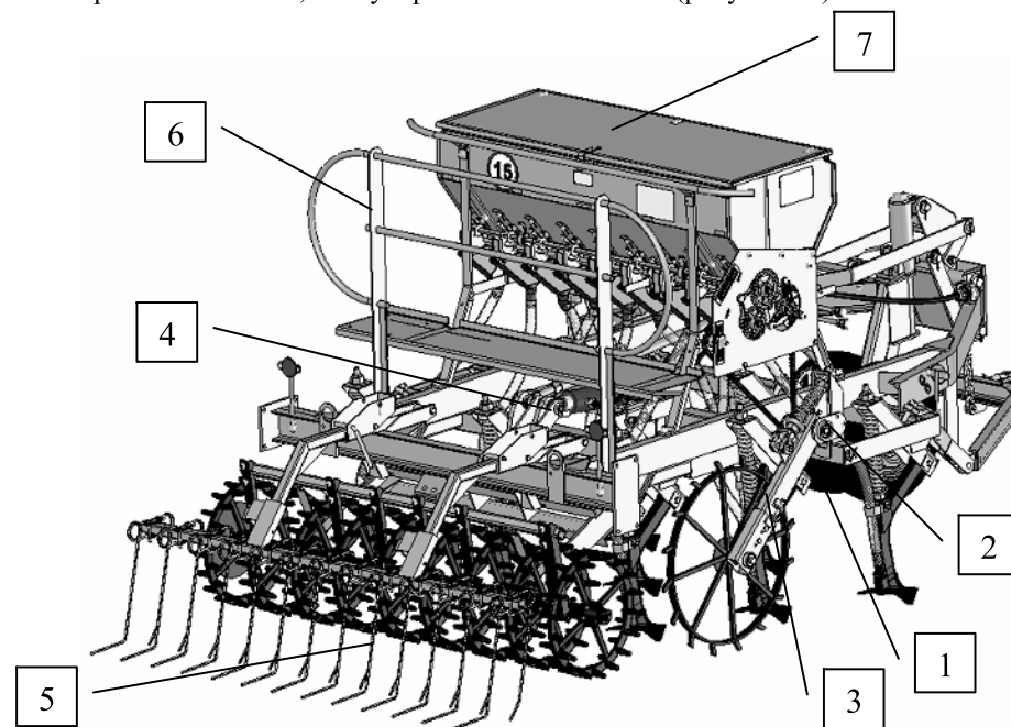
Рисунок 47- Сеялка СКП-2,1К
