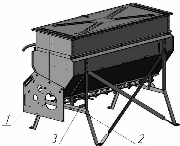
Рисунок 41 -Ящик зернотуковый увеличенной ёмкости с укороченной боковиной
