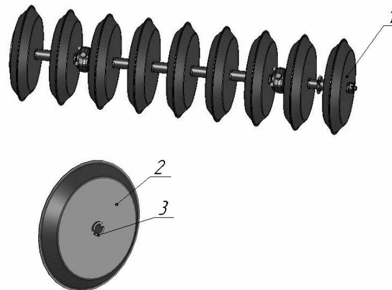
Рисунок 386- Батарея катков с клиновыми катками СКП 01.23.000Л
