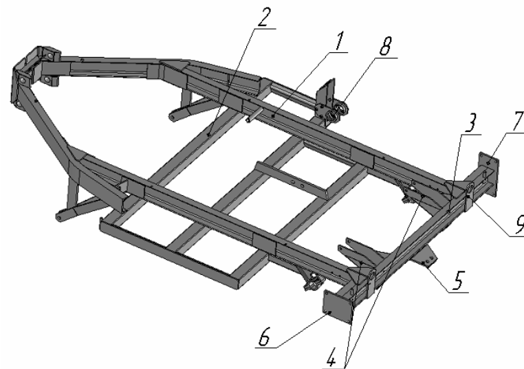
Рисунок 40 - Рама СКП 01.01.000М-02
