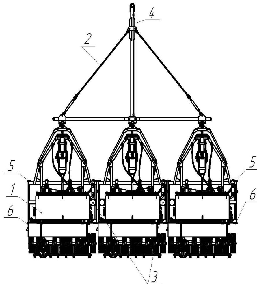
Рисунок 20- Посевной комплекс КСКП 2,1 х3
