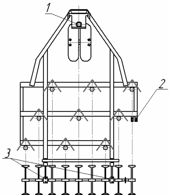
Рисунок 56- Схема смазки Сеялок СКП-2,1И; СКП-2,1К
