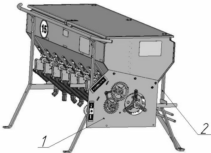
Рисунок 48 – Ящик зернотуковый с укороченной боковиной СКП 01.13.000В
