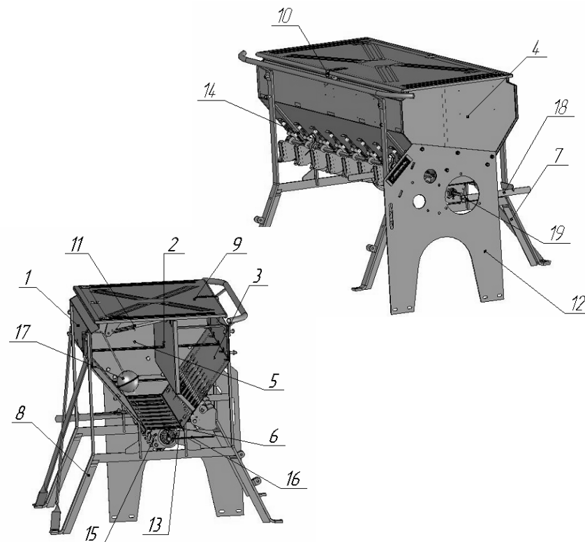
Рисунок 6- Ящик зернотуковый СКП 01.13.000
