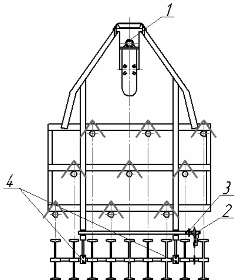
Рисунок 25- Схема смазки
