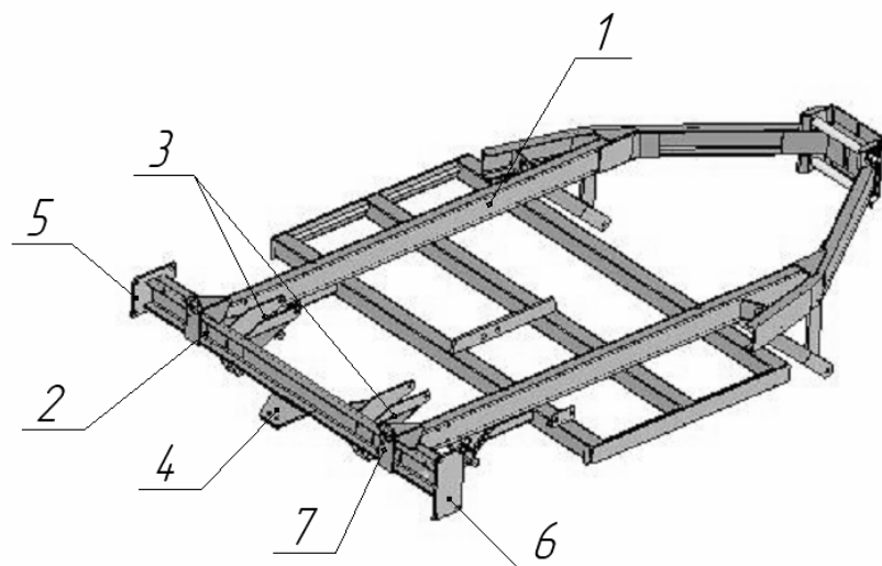
Рисунок 486 – Рама СКП 01.01.000ВД
