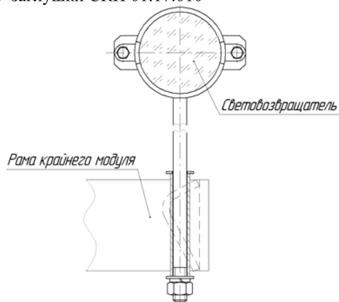
Рисунок 22- Крепление световозвращателя
