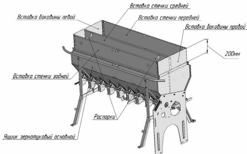
Рисунок 30- Комплект для наращивания зернотукового ящикаСКП-КТ№14 (для запчастей)
