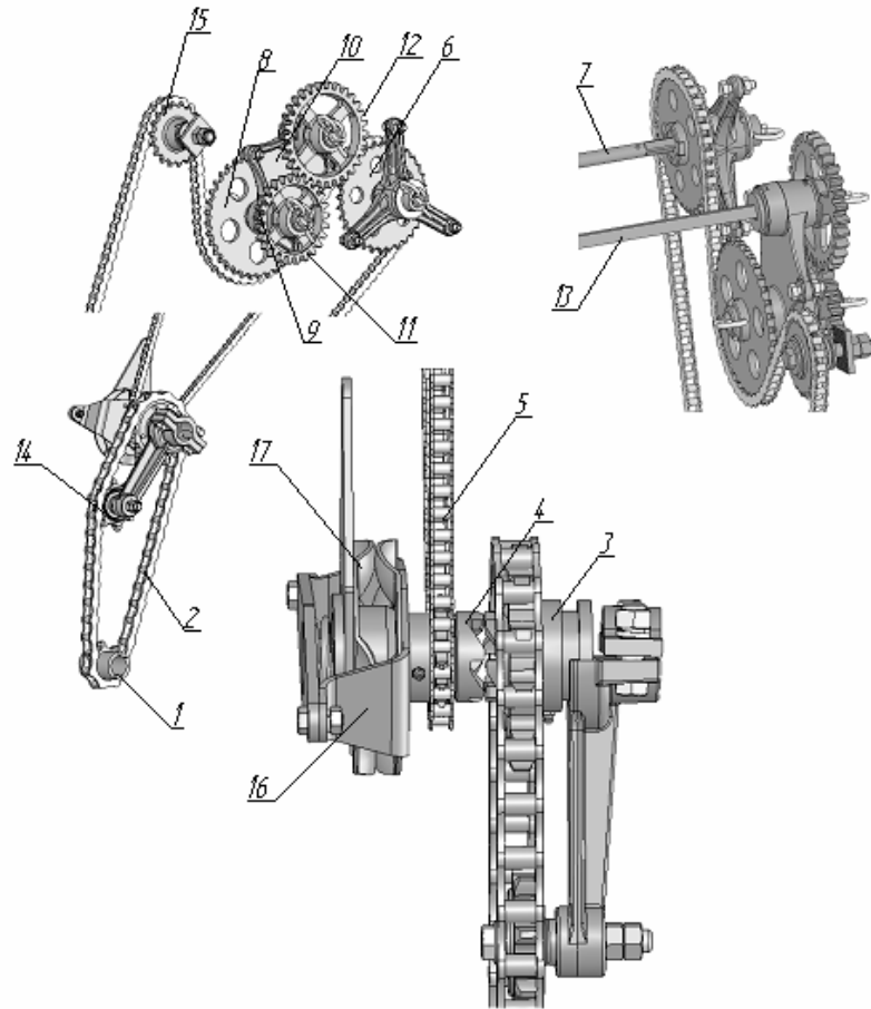
Рисунок 12- Механизм привода СКП 01.06.000А
