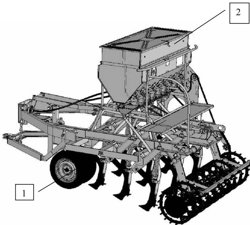
Рисунок 28- Сеялка СКП-2,1Б
