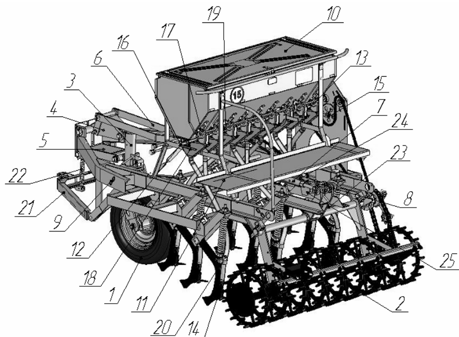
Рисунок 1-Сеялка СКП-2,1
