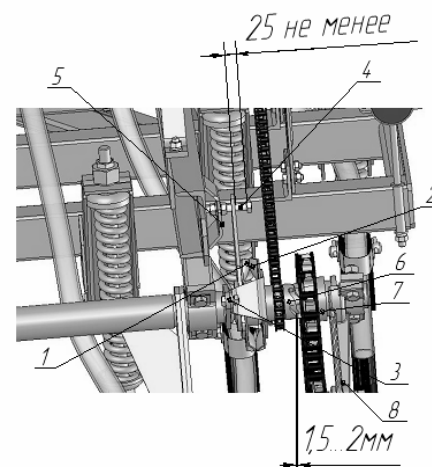
Рисунок 17 Регулировка механизма включения и выключения высевающих аппаратов.
