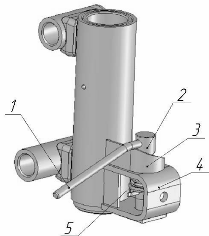
Рисунок 5- Фиксатор
