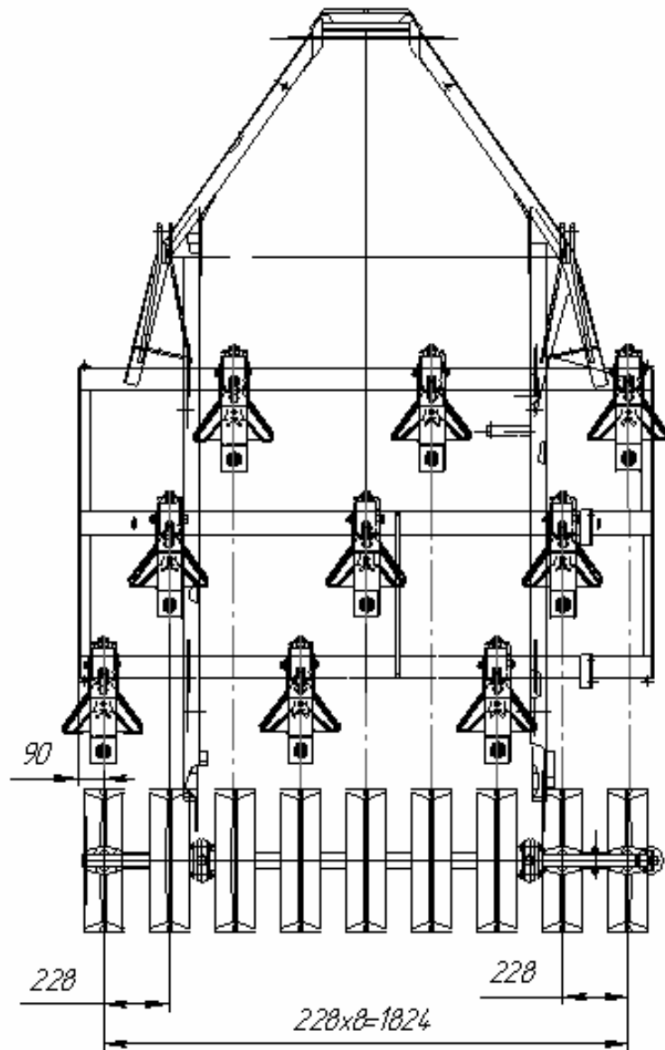
Рисунок 19- Схема расстановки сошников
