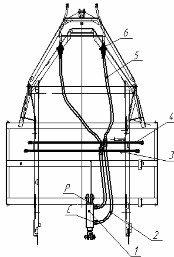
Рисунок 15- Гидросистема сеялки
