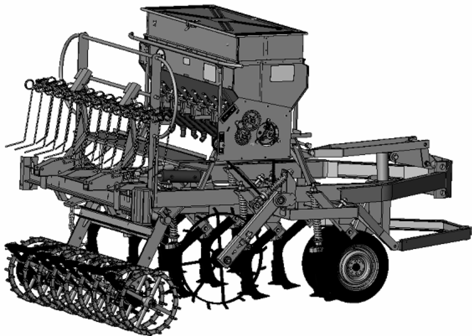
Рисунок 44- Транспортное положение бороны пружинной
