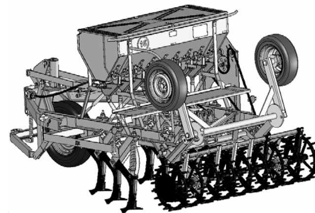
Рисунок 32- Рамка колёсная в рабочем положении
