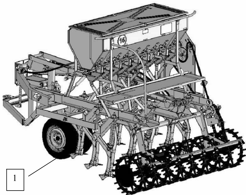
Рисунок 26- Сеялка СКП-2,1А
