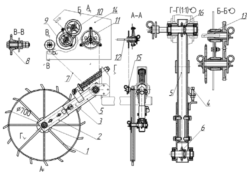
Рисунок 46- Схема независимого привода
