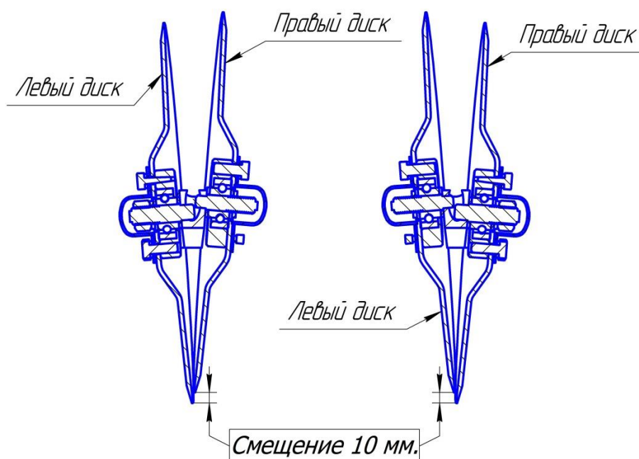
Задний сошник
