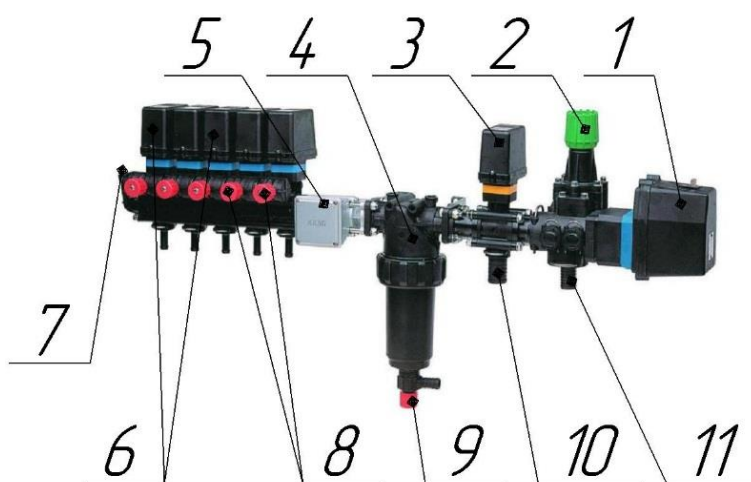
Рис. 9. Электромеханический регулятор-распределитель
