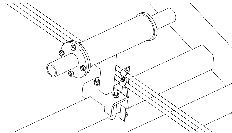
Рис.9 Амортизатор.
