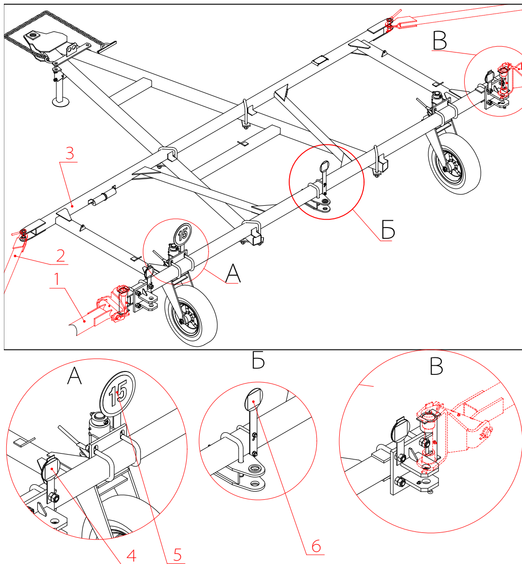
Рис. 15а. Перевод сцепки в транспортное положение (с частичной разборкой) при транспортировке по дорогам общего пользования. 1- Балка боковая СП11К 01.030/040; 2- Растяжка СП11К 01.050; 3- Секция центральная СП11К 01.010; 4-Световозвращатель СП16К 00.170А; 5- Знак ограничения скорости СП16К 00.180; 6- Светоотражатель красный.
