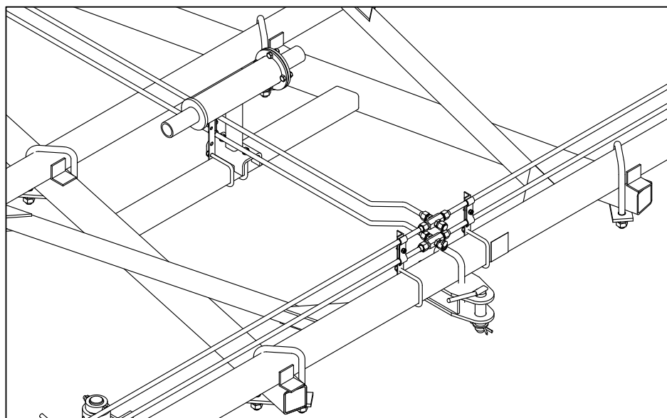
Рис.12 Крепление дышла к центральной секции.
