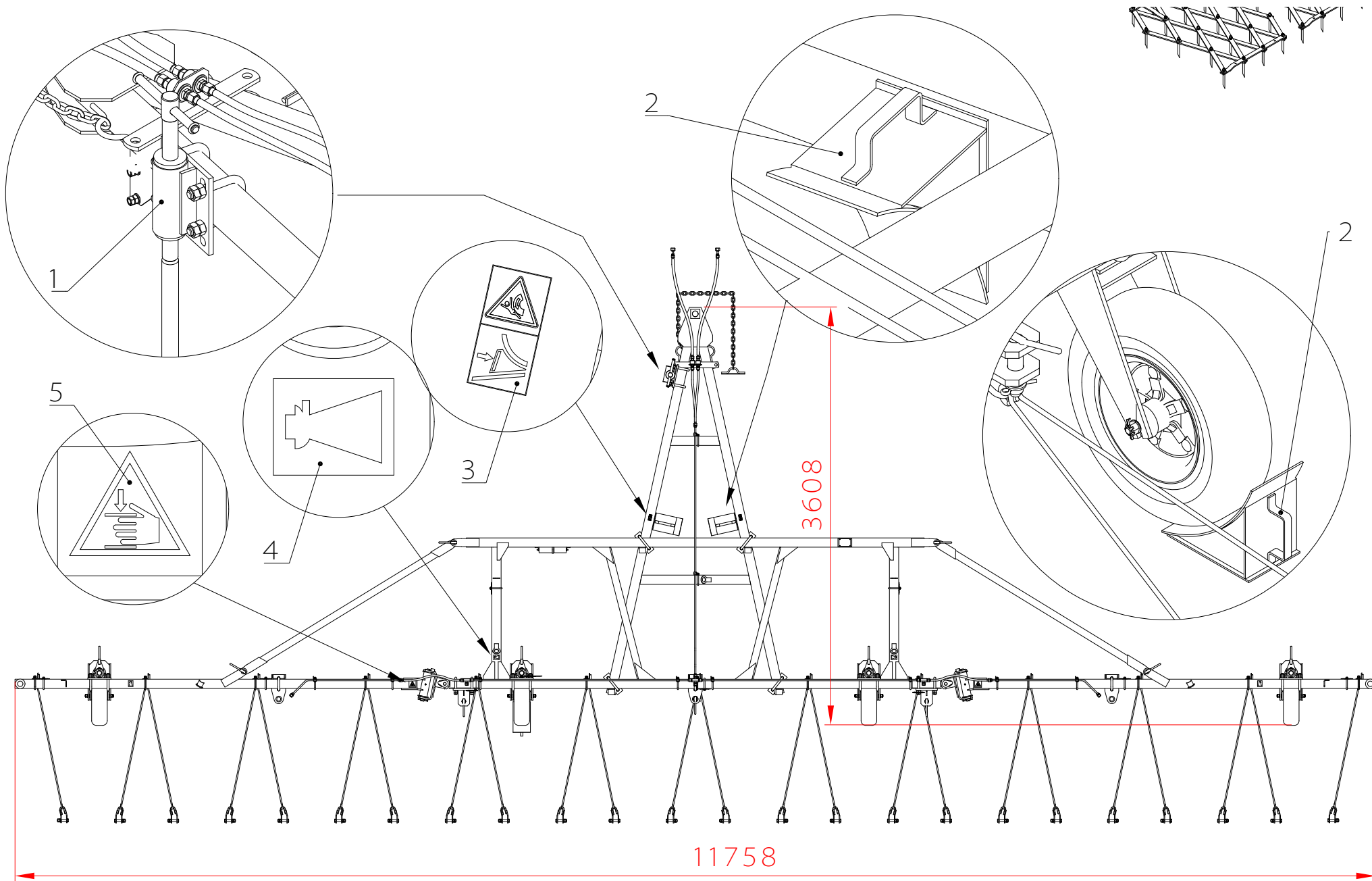
Рис.2а Сцепка в сборе 1- Опора транспортная СГ21К 00.070; 2- Противооткатный упор КИР 00.020; 3- Место закрепления противооткатных упоров; 4- Место установки домкратов; 5- Опасное защемление рук
