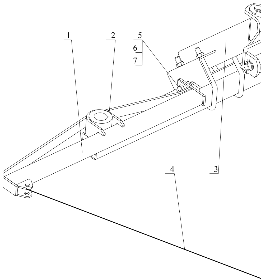
Рис.7 Установка кронштейна цепи. 1- Кронштейн цепи; 2-Посадочная втулка балки; 3-Кронштейн маркера; 4-Тросовая растяжка; 5-Болт М16х35; 6-Гайка М16; 7-Шайба 16.65Г
