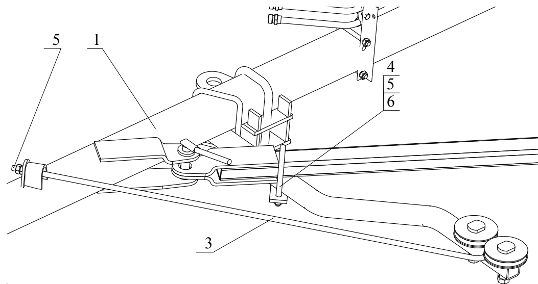
Рис.8 Кронштейн роликов. 1-Балка; 2-Растяжка; 3-Тяга; 4-Скоба; 5-Планка; 6-Гайка М12
