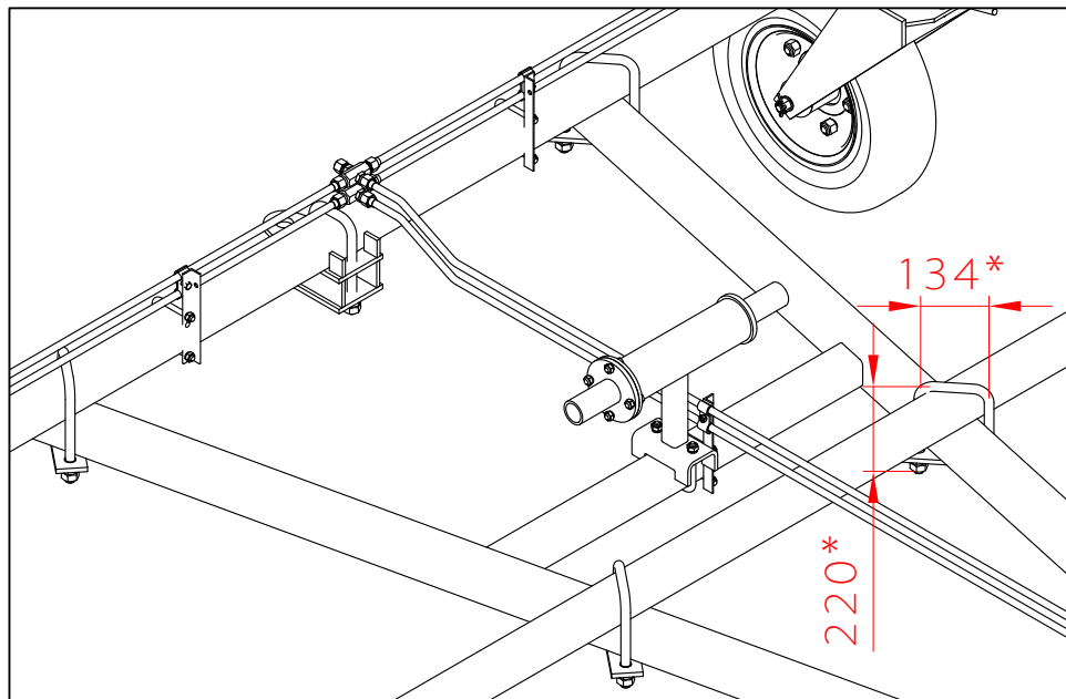
Рис.12 Крепление дышла к центральной секции.
