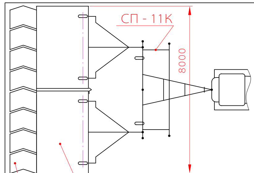
Рис. 14 Схема агрегирования сцепки с культиваторами (рабочее и транспортное положение)
